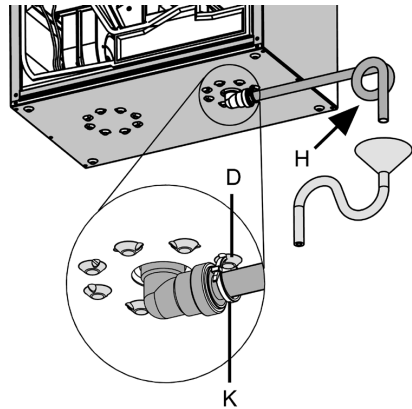
Abbildung: Lüftungsgerät in Rechtsausführung, Linksausführungen spiegelt sich
